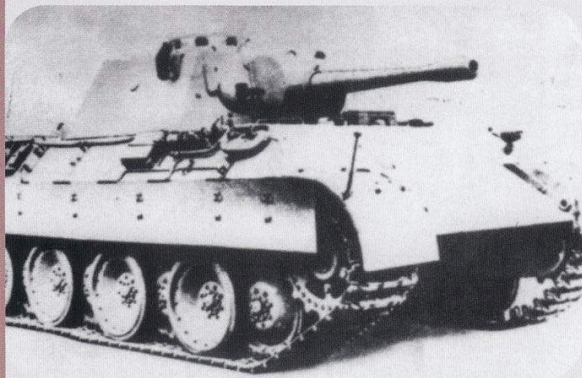
7230 Pz.Beob.Wg. V Ausf. G
